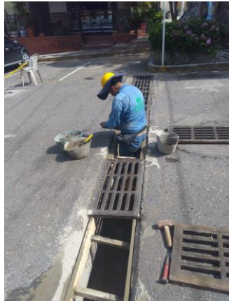
ARREGLO DE PESTAÑAS CASTILLA REAL I
